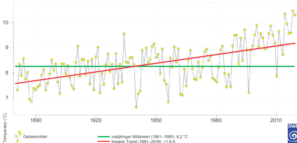
Grafik 1: Jährliche mittlere Temperaturen und linearer Trend in Deutschland 1881–2019 (Quelle: DWD)
