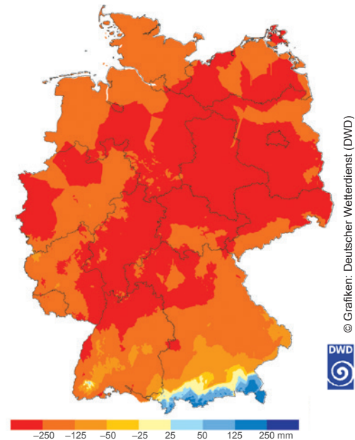
Grafik 2: Klimatische Wasserbilanz 01.06.–31.08.2018 (Quelle: DWD)
